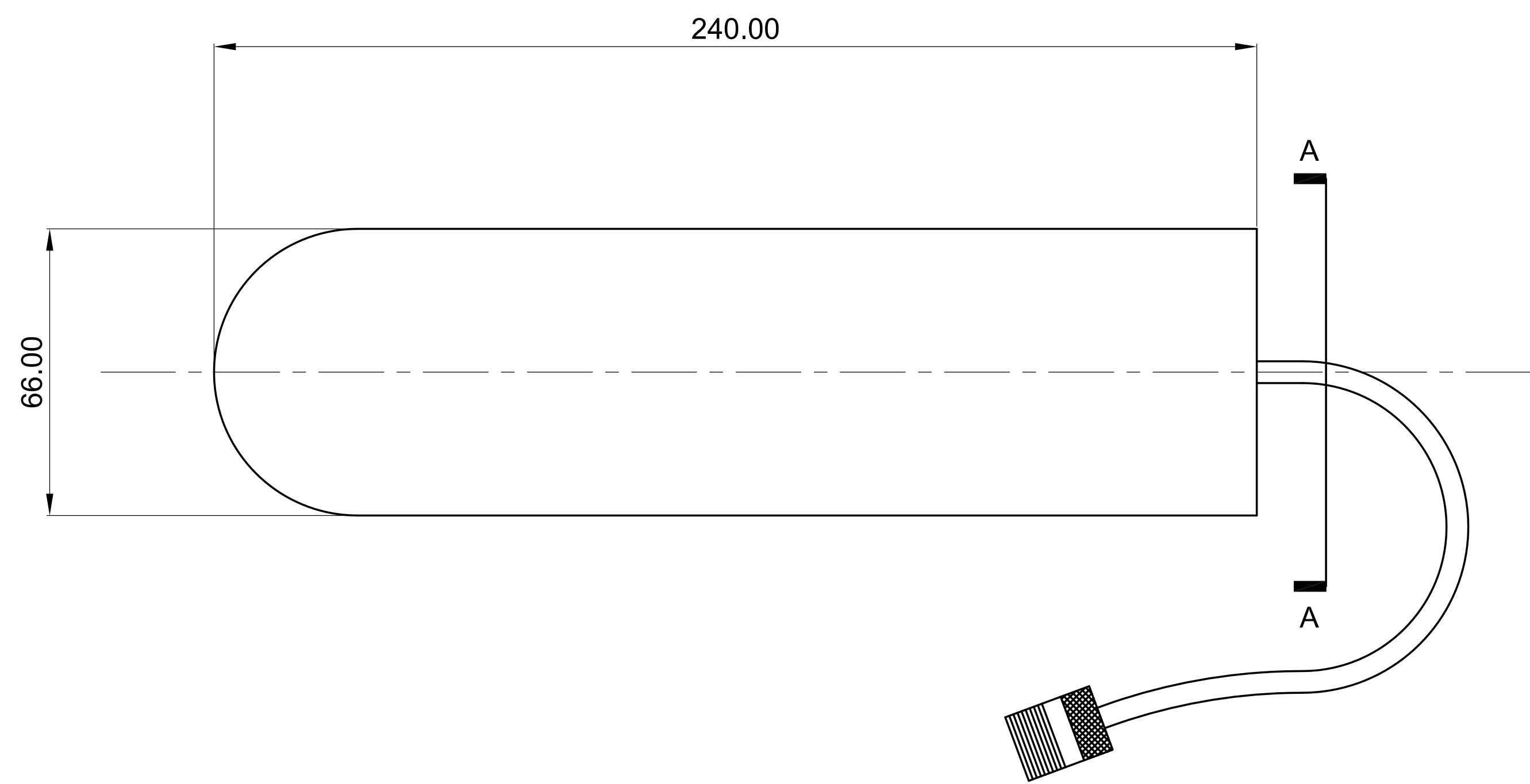
ANTENNA
